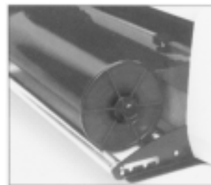
Abb.: 2: Folienführung mit Flanschen
